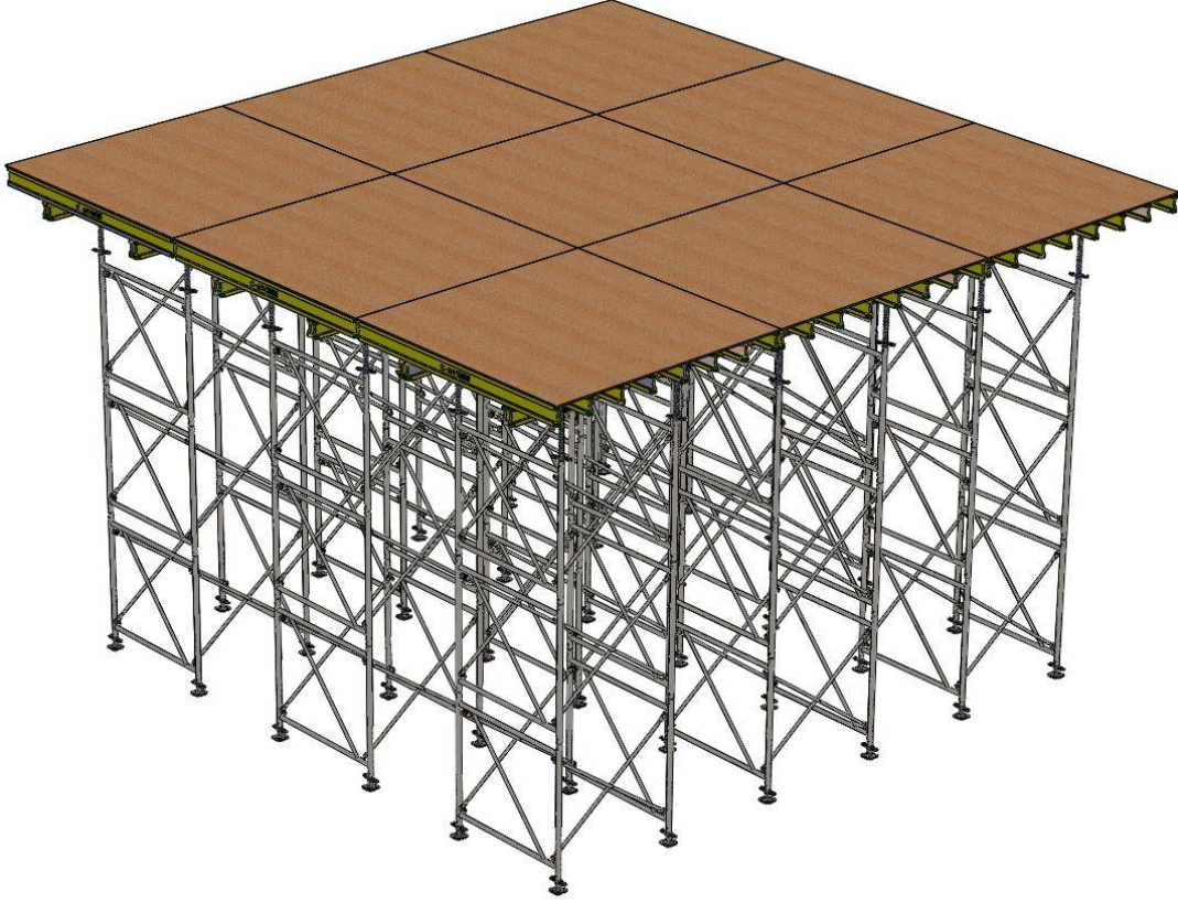
Şekil 4.6. Kalıp altı ağır yük iskelesi’Masa tip iskele sistemi yerleşim örneği
