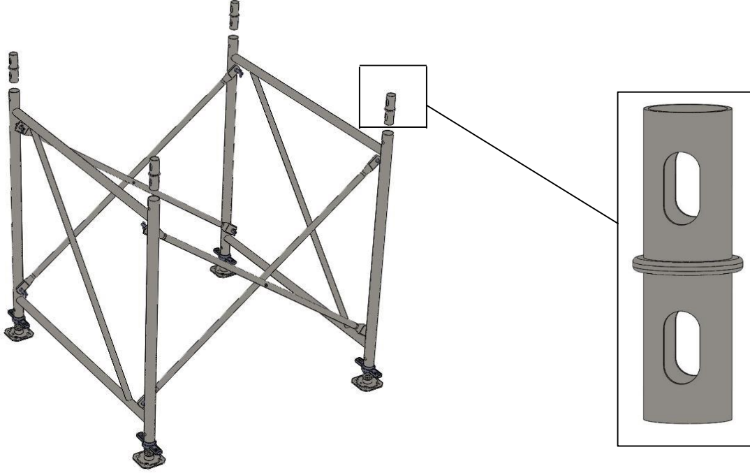
Şekil4.3. Çerçeve ekleme elemanlarının montajı
