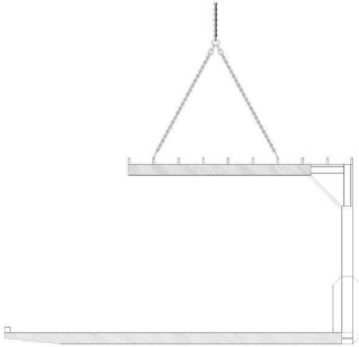
Şekil 5.4. Masa taşıma çatalı örnek tip kesiti
