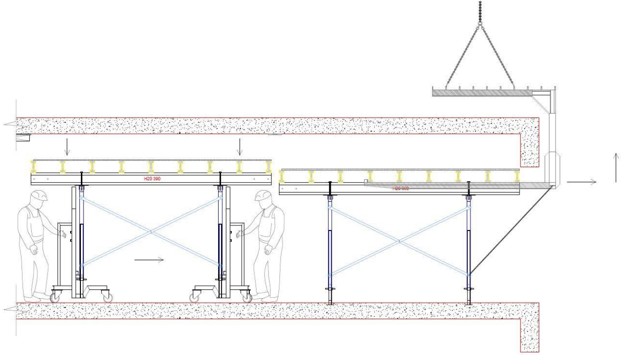
Şekil 5.3. Kiriş alt kotuna indirilen masa kalıbının masa taşıma çatalı vasıtasıyla bir üst kata taşınması
