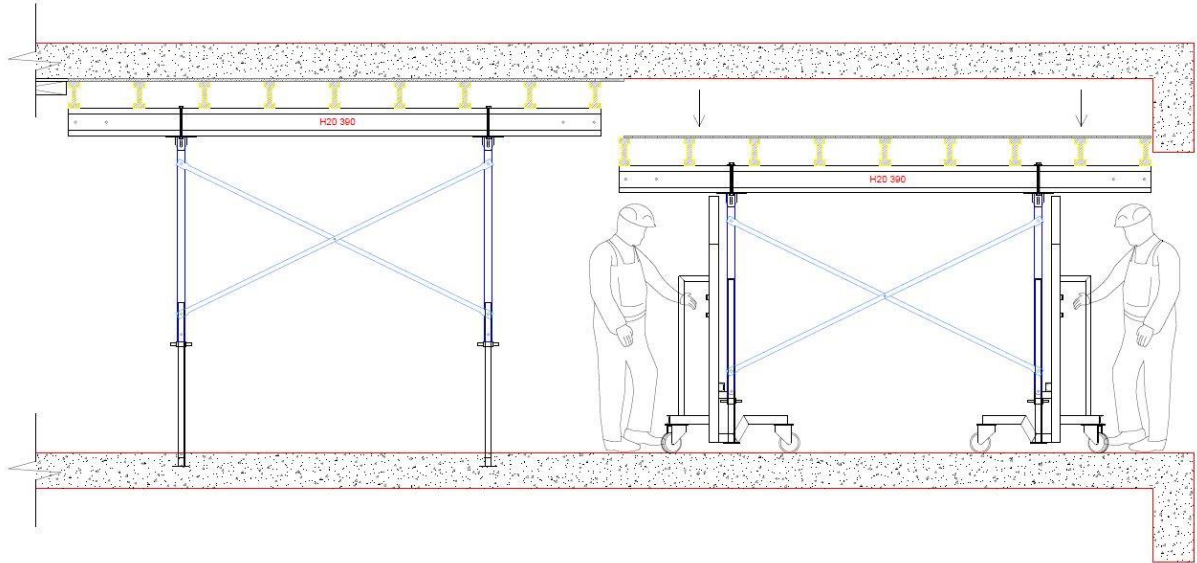
Şekil 5.2. Masa taşıma arabası vasıtasıyla kalıbın indirilmesi
