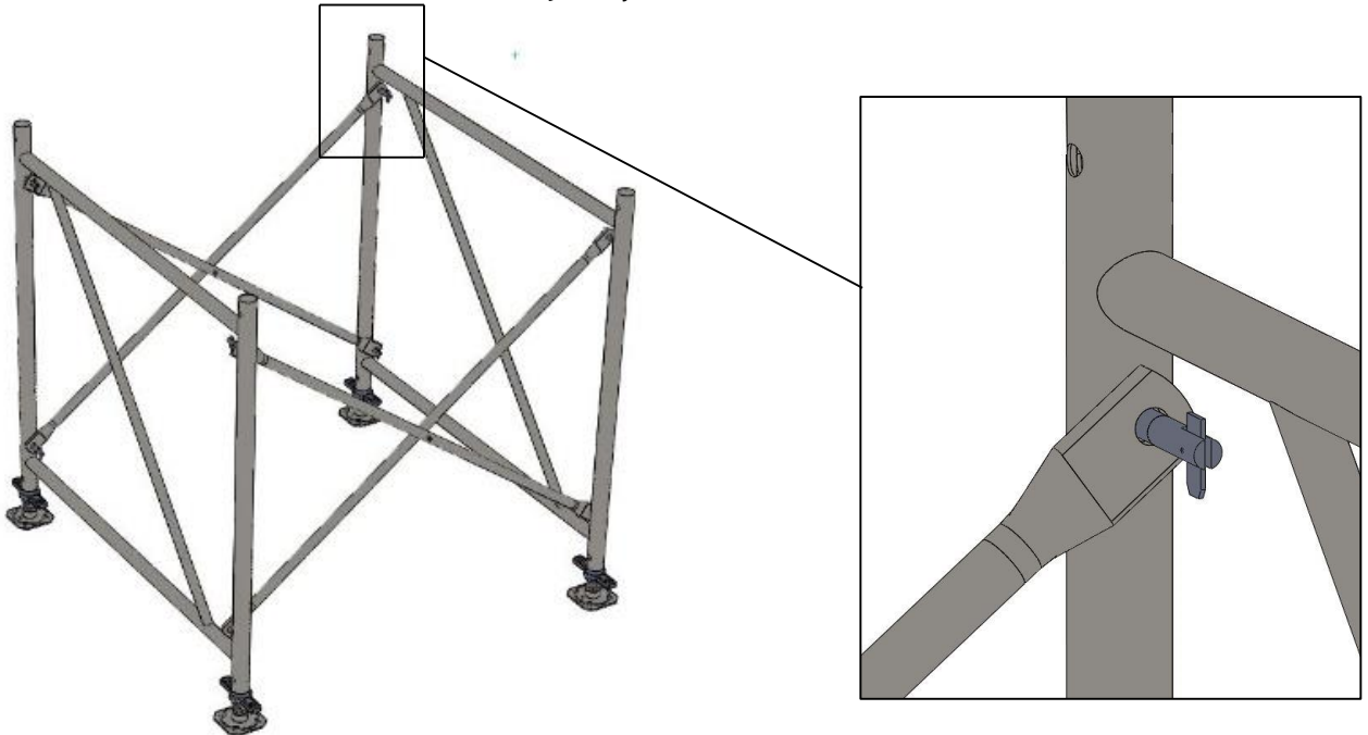
Şekil4.2. Çerçeve elemanlarındaki pimlere çapraz elemanların montajı
