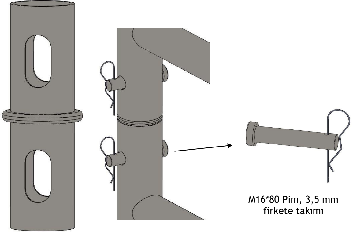
Çerçeve ekleme elemanına pim-kopilya bağlantısı
