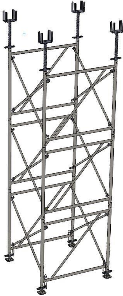
Şekil4.4. Üst kat çerçevelerinin montajı, 4 yollu başlık üst ayar millerinin montajı.
