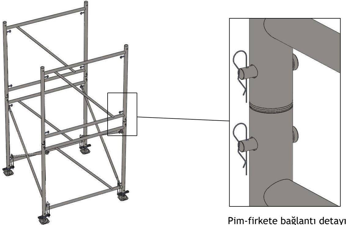
Şekil4.3. Çerçeve ekleme elemanlarının montajı
